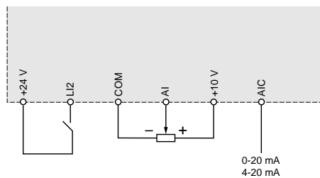
Wiring schematic
